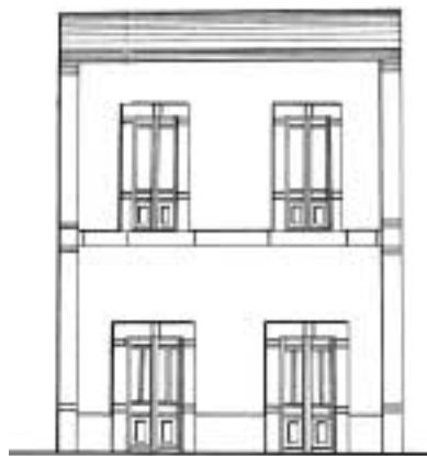
Dibuix de façana de la central elèctrica
