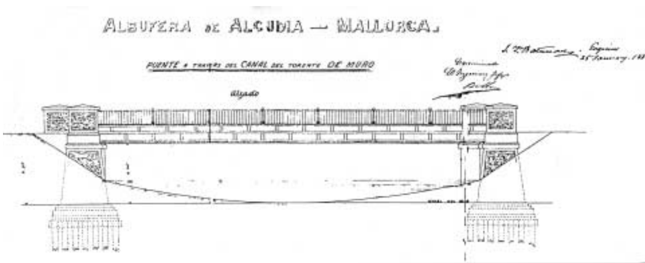
Pont de Son Carbonell. Dibuix original de J. F. Bateman. DA: 150 anys d'obres públiques a les Illes Balears, Sa Nostra, Palma 1996
