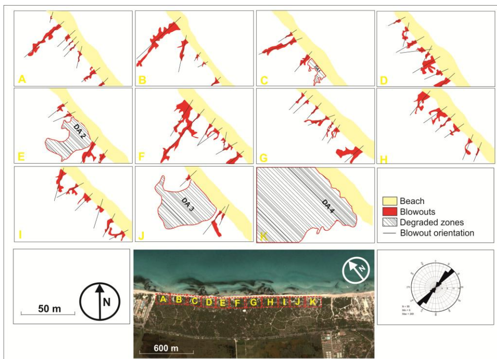
Fig. 9. Orientació dels blowouts analitzats. Platja d'es Comú de Muro.
