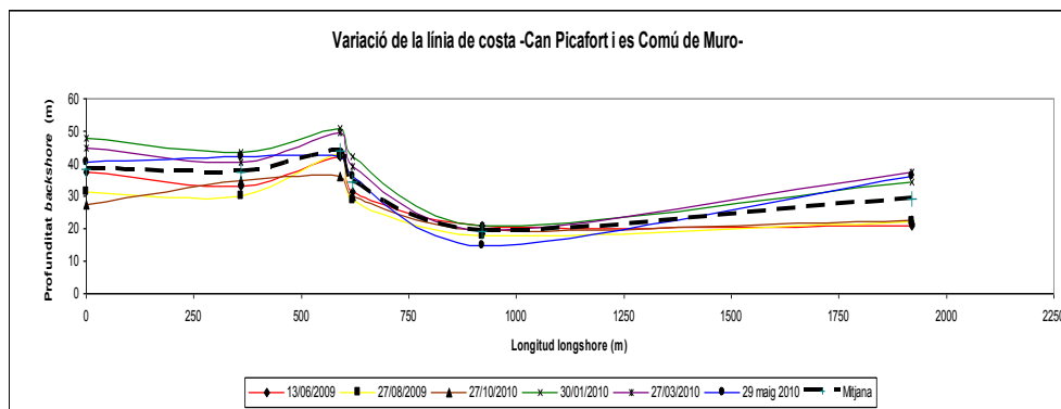
Fig. 4. Representació gràfica de la variació anual de la línia de costa en el sector estudiat.
