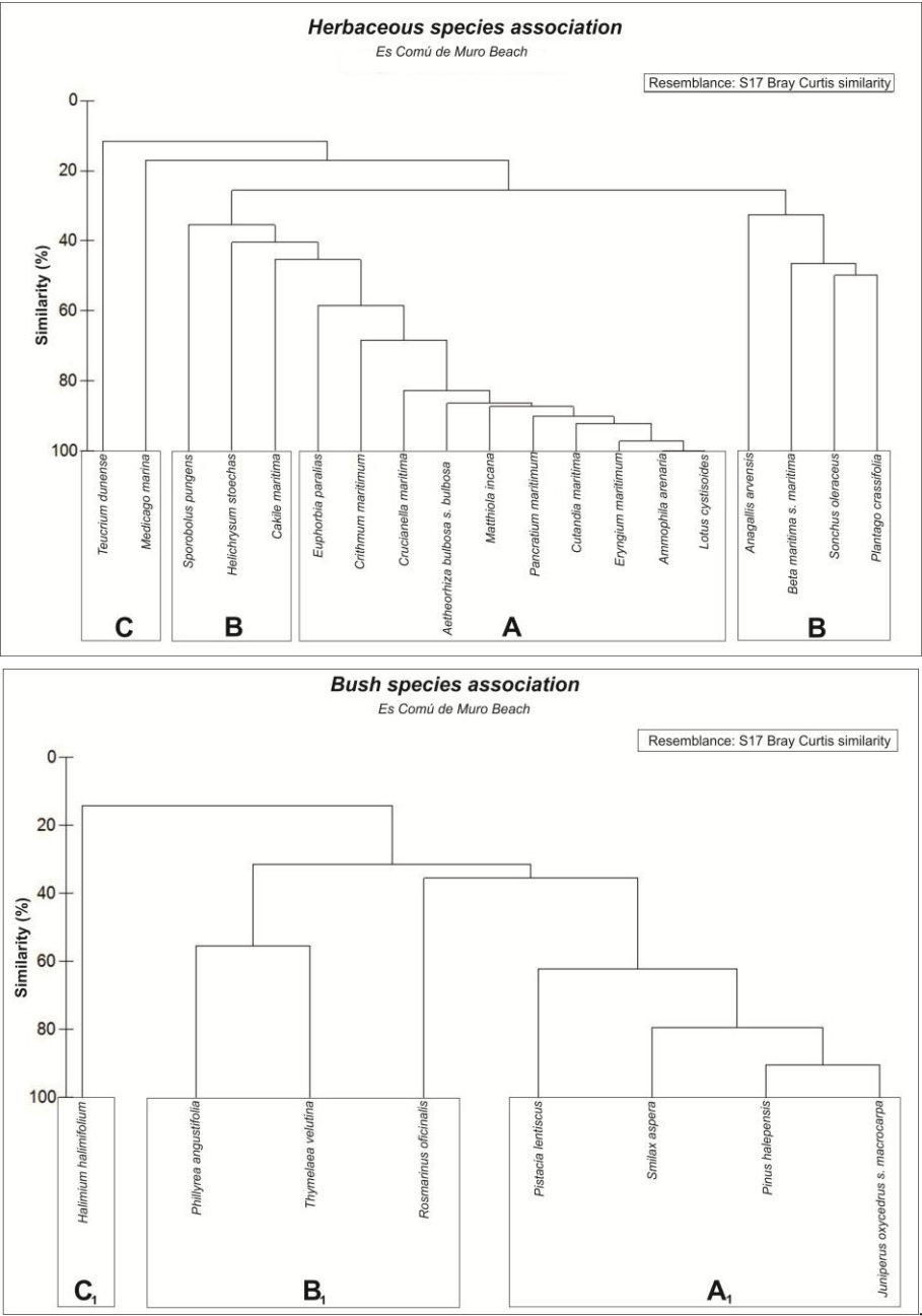
Fig. 12. Anàlisi cluster de les espècies herbàcies (superior) i llenyoses (inferior) analitzades.
