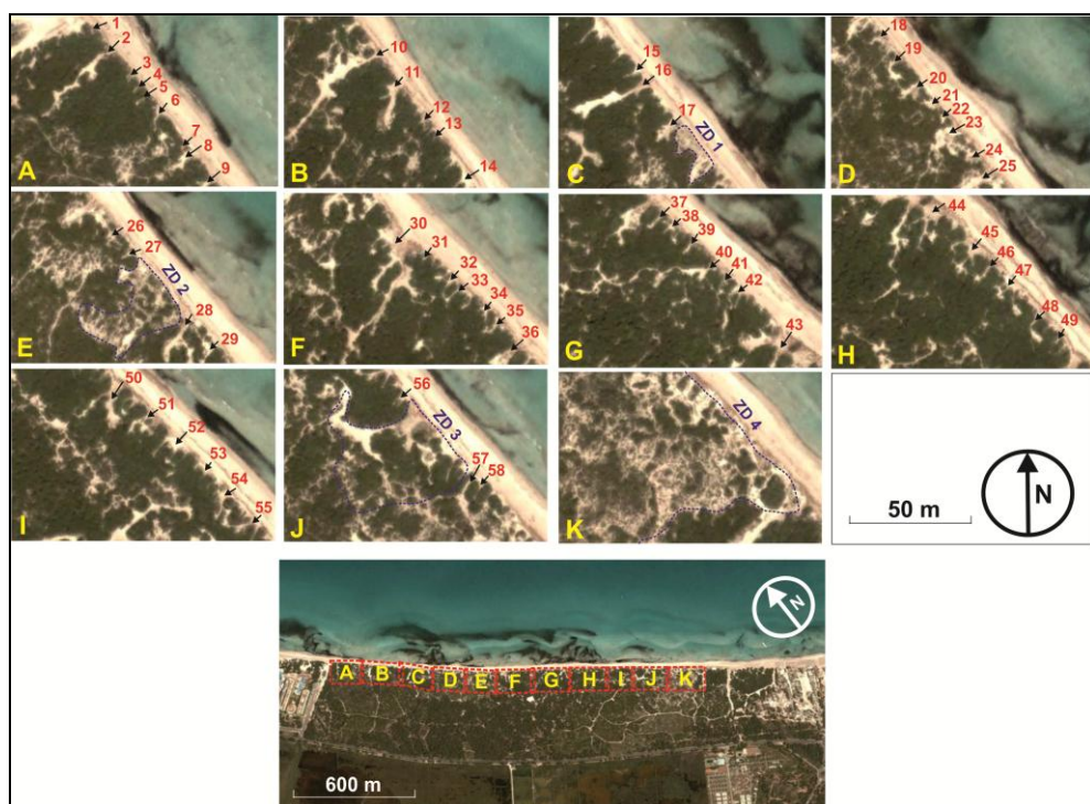
Fig. 8. Localització dels blowouts analitzats. Platja d'es Comú de Muro.
