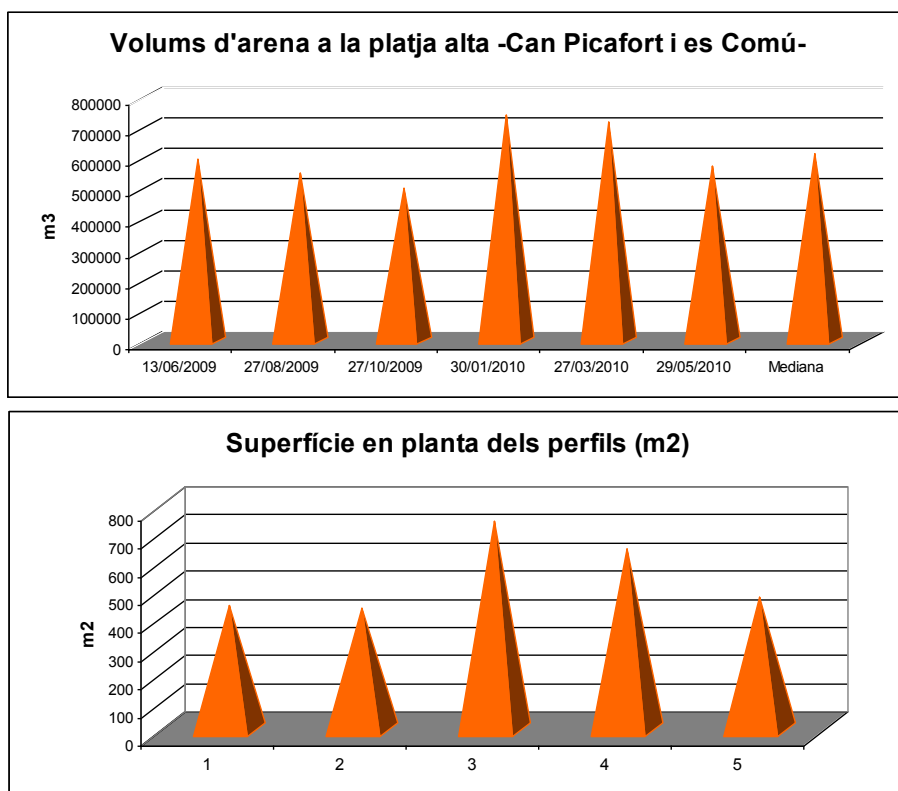
Fig. 7. Volums sedimentaris per dies de mostreig.
