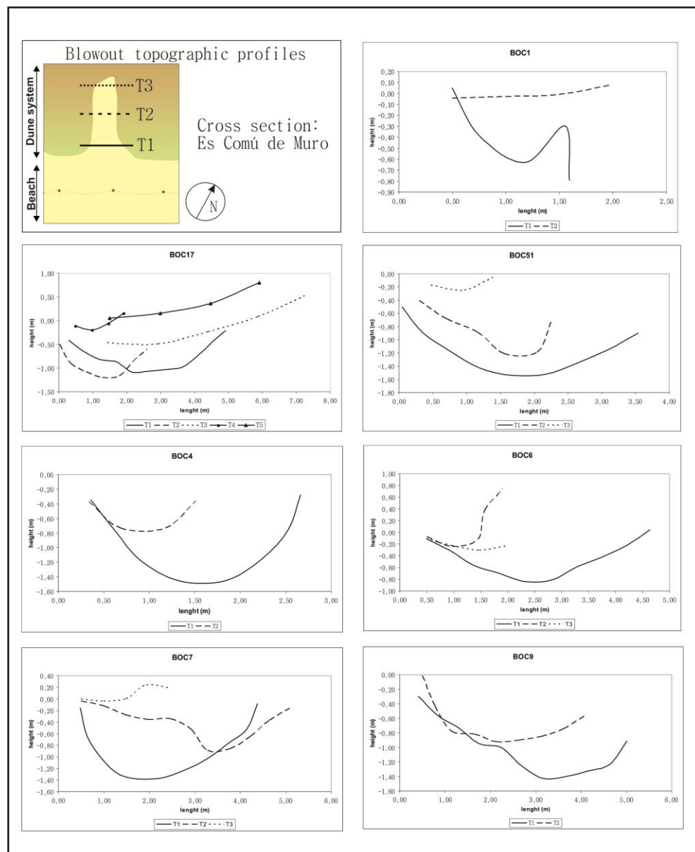
Fig. 10. Alguns exemples representatius de perfils topogràfics interns.
