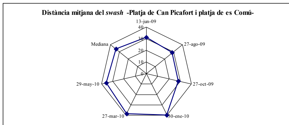
Fig. 5. Representació de la distància del punt d'swash per cada dia de mostreig.
