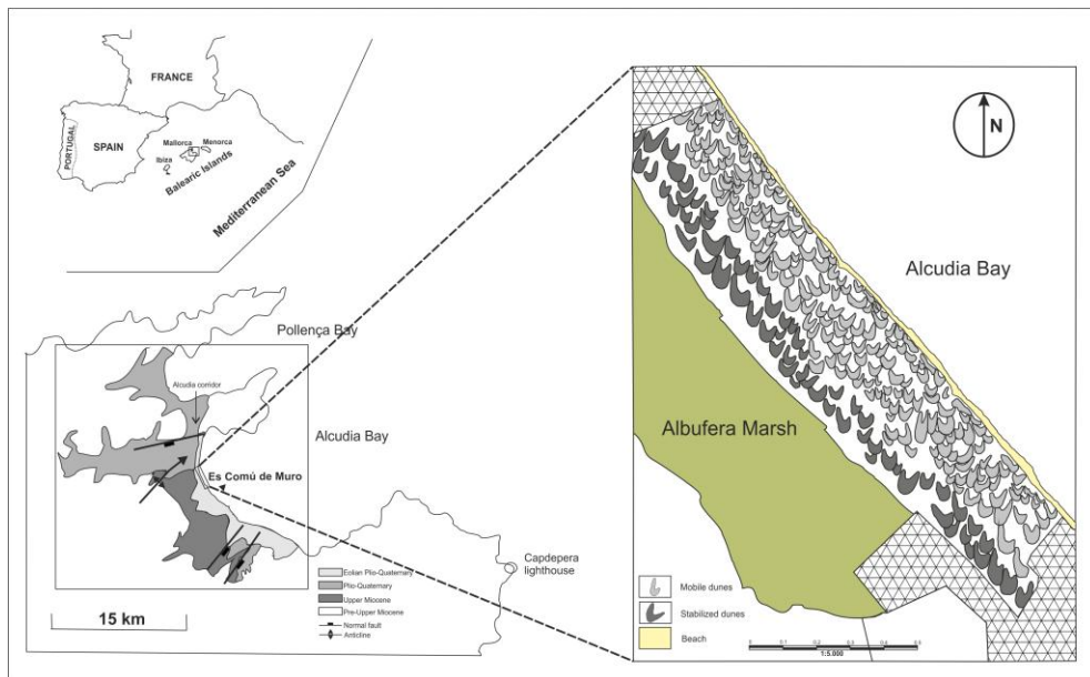
Fig. 1. Localització de la zona d'estudi i esquema geomorfològic del sistema dunar.
