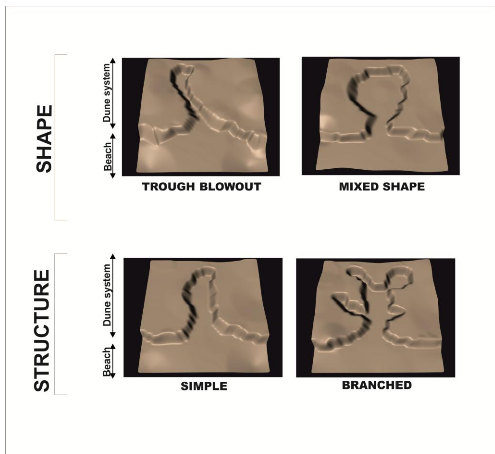
Fig. 11. Classificació morfomètrica dels blowouts a partir de la seva forma i estructura.
