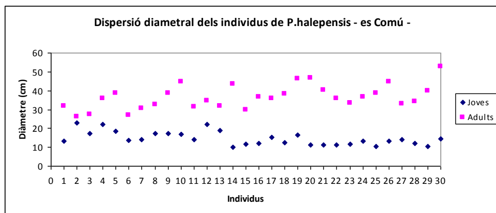
Fig. 13. Diferència de diàmetre entre els individus de P. halepensis mostrejats.
