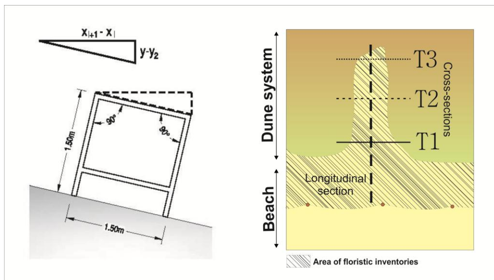
Fig. 3. Esquema del pantòmetre. A la dreta, localització dels perfils topogràfics realitzats.
