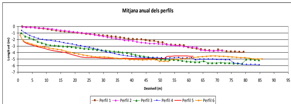
Fig. 6. Representació gràfica dels perfils mitjans anuals a la platja de Can Picafort i es Comú de Muro.
